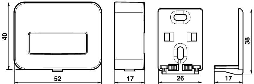
Abbildung 1: Dimensions in mm
